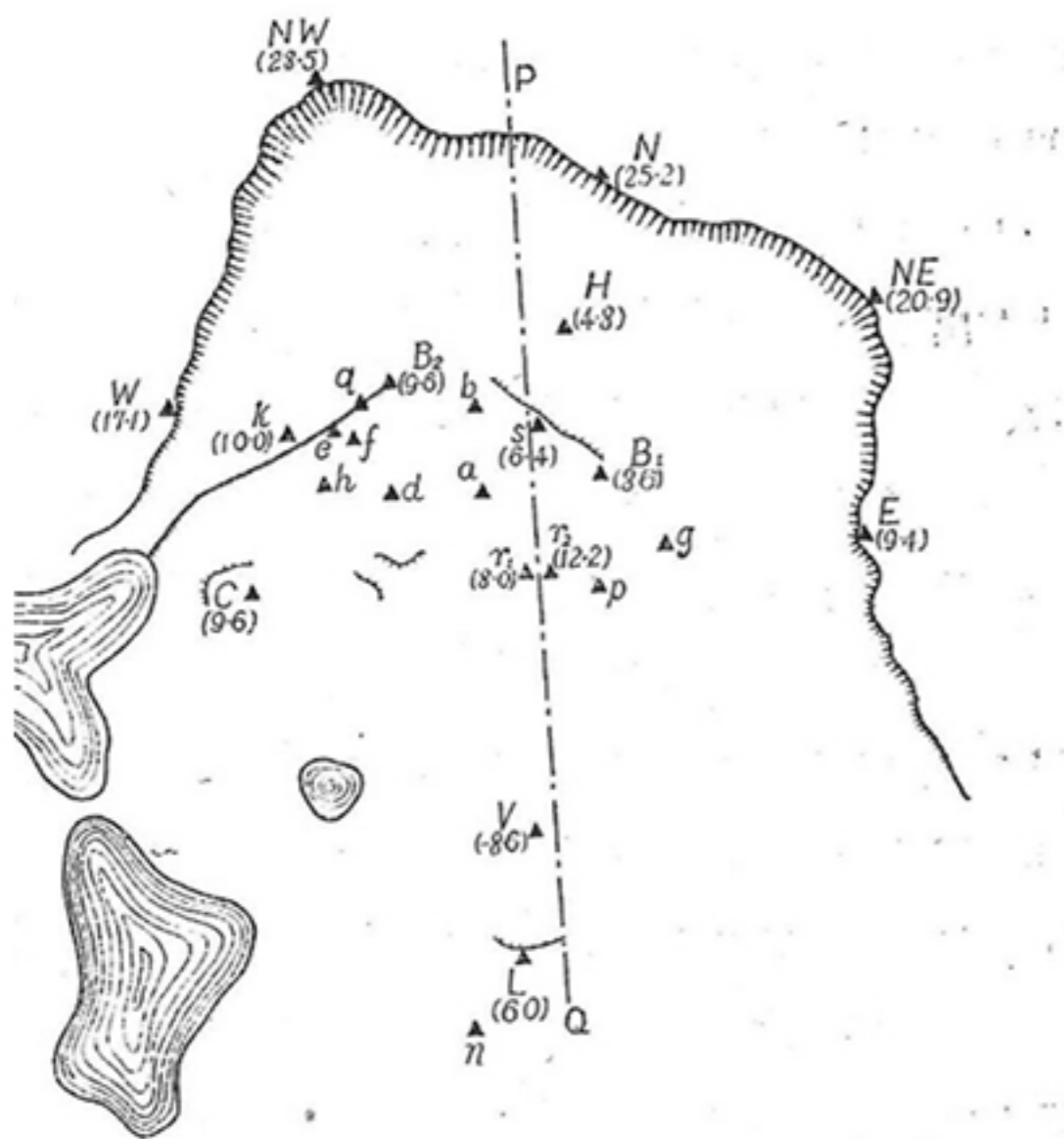
図9 震生湖の崩壊地の実測平面図 (▲は平板測量の実測平面図) (図9, 図10とも寺田・宮部, 1932)
