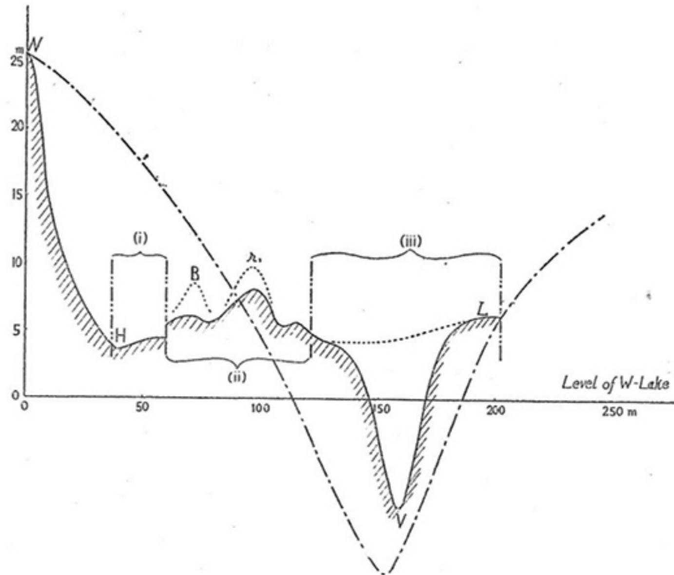
図10 図9におけるP-Qの断面図 (一点鎖線は地震前の谷のプロファイルを示す)
