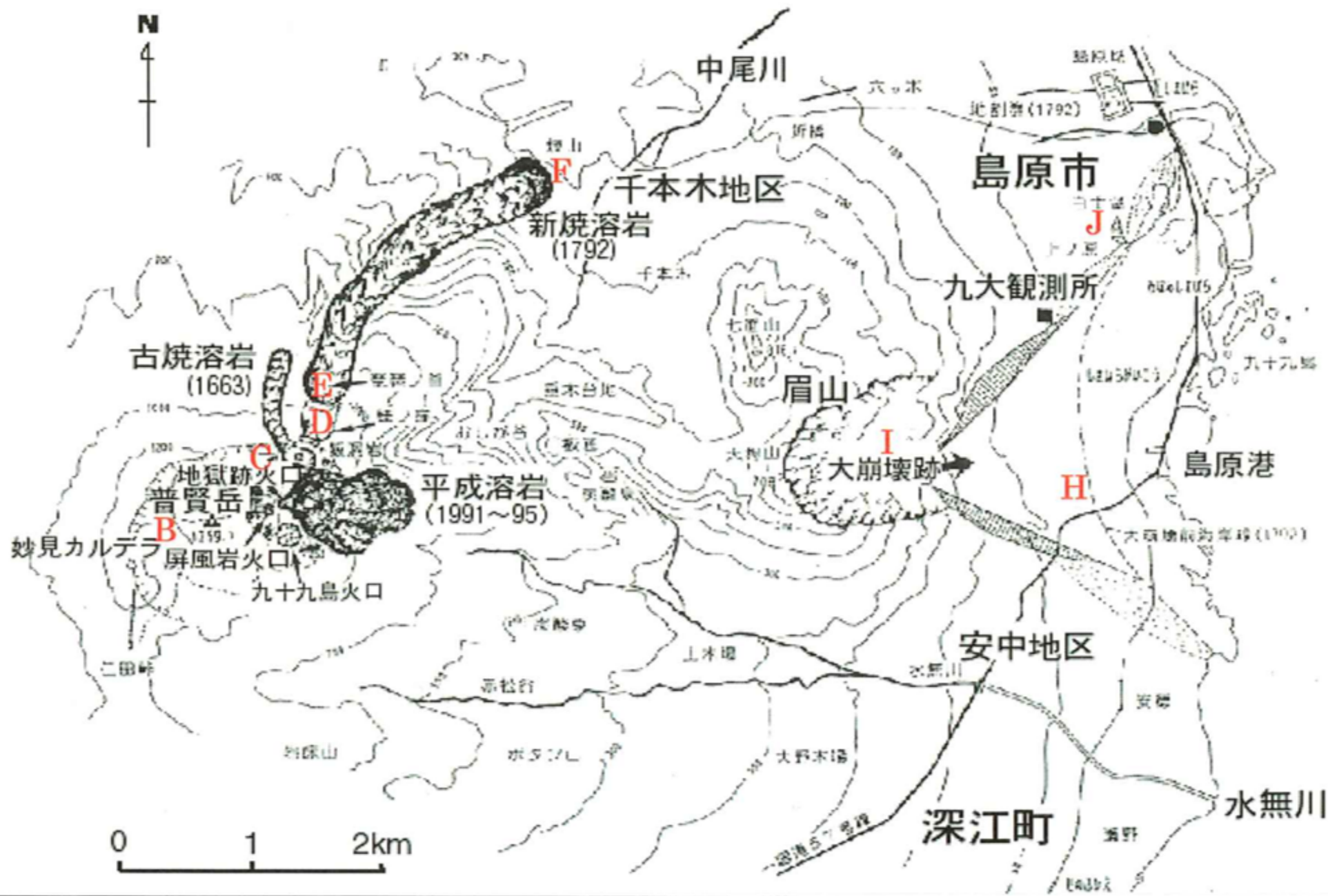
図 3.2 雲仙普賢岳と眉山，噴火位置の推移（太田（1984）をもとに井上（1999）追記
