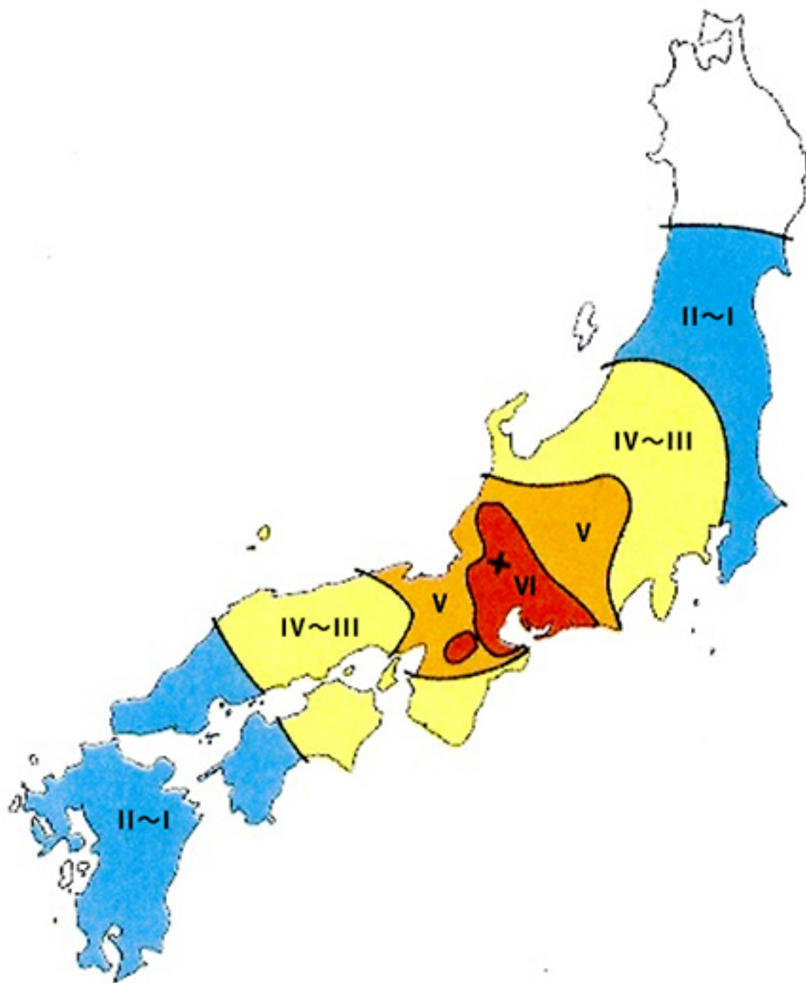
図4 濃尾地震の震度分布 (気象庁, 1983)
