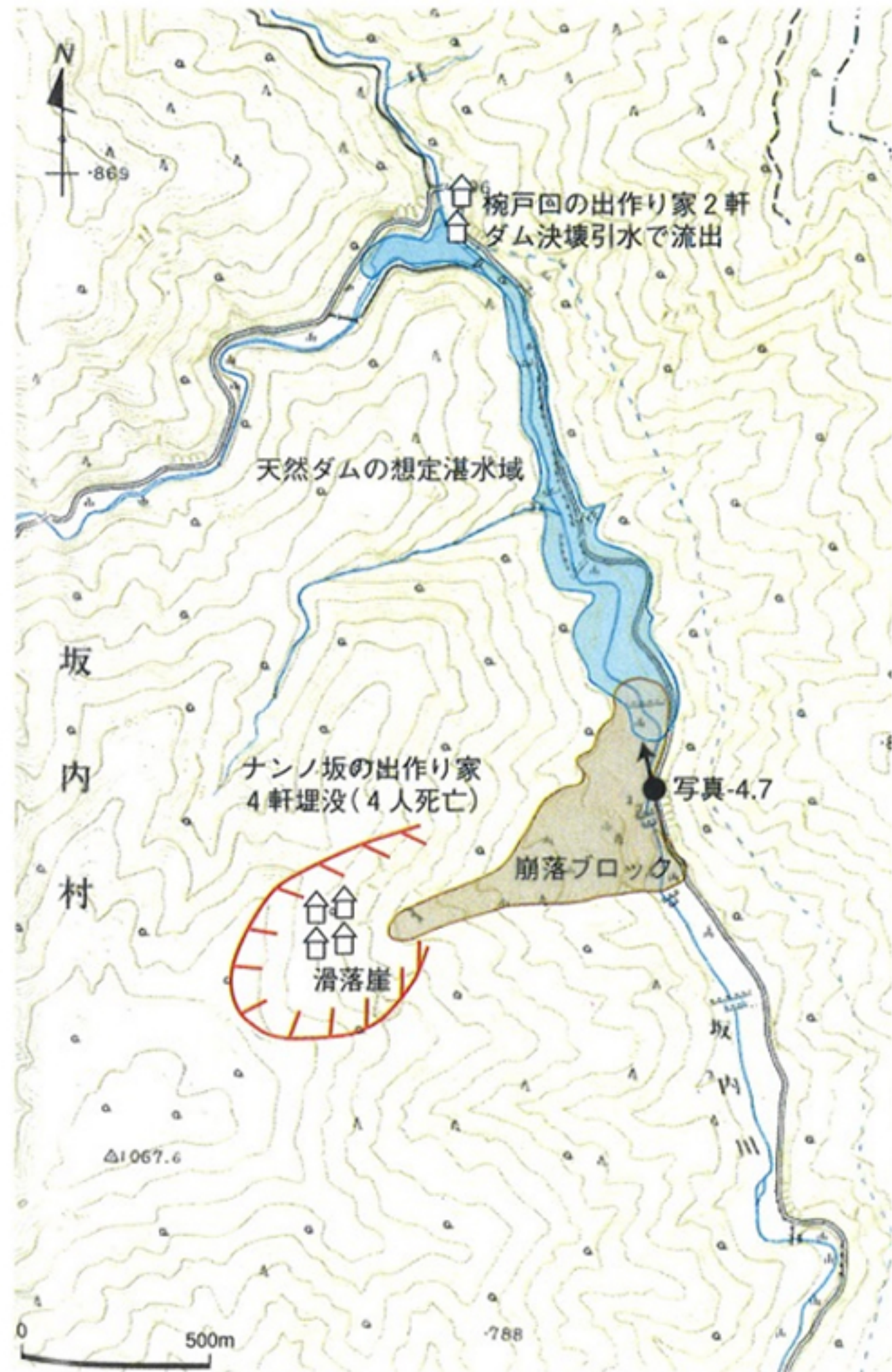
図9 ナンノ崩壊の土砂災害状況図
