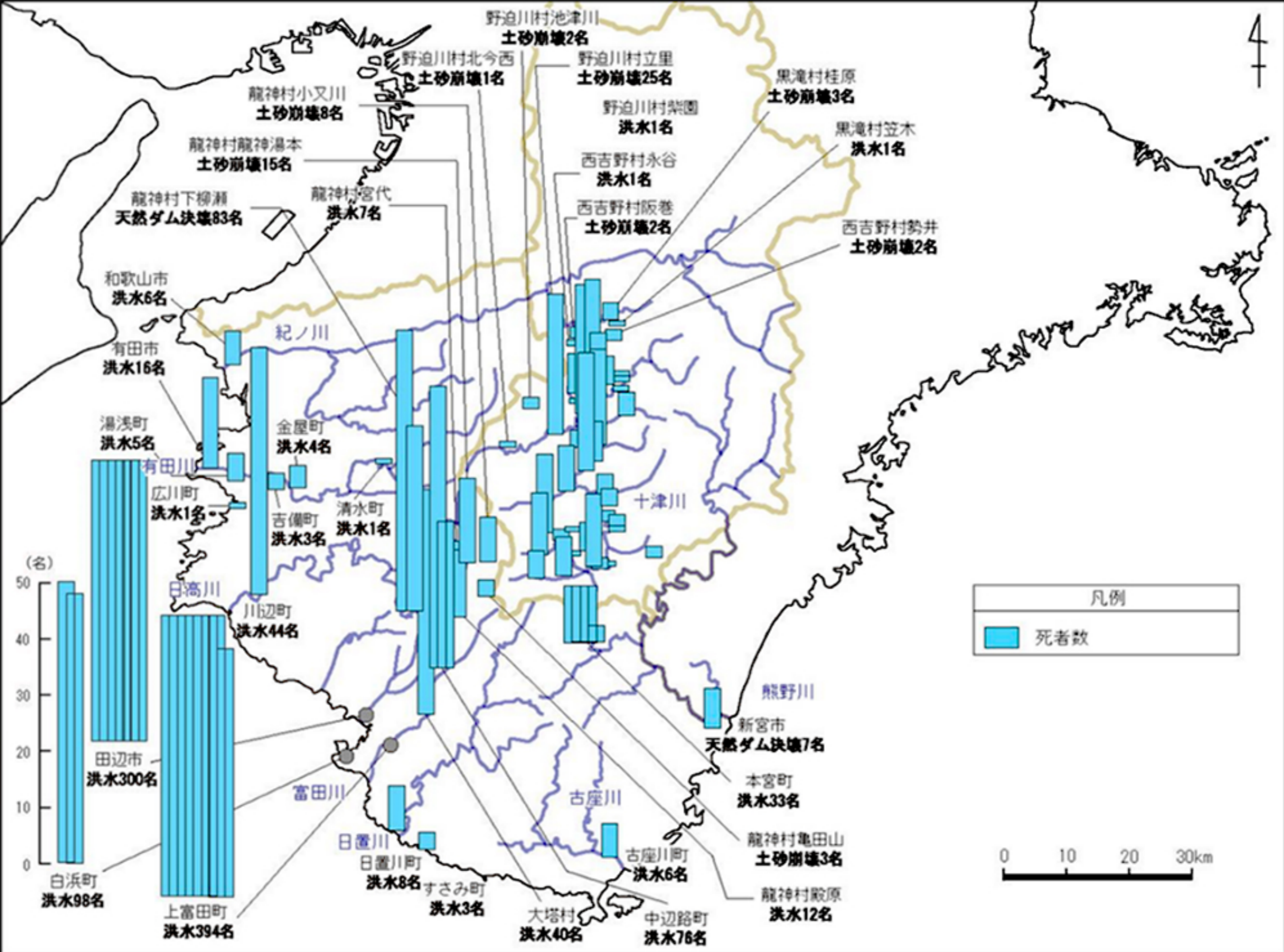
図 1 1889 年紀伊半島災害による和歌山県と奈良県における死者数 (水山ほか, 2011; 明治大水害誌編集委員会, 1989 をもとに作成; コラム 28, 85)
