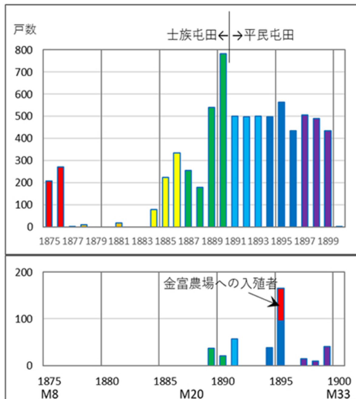
図5 年次別屯田兵入殖戸数 (下段は和歌山県からの入殖者, 酒井利啓作成)
