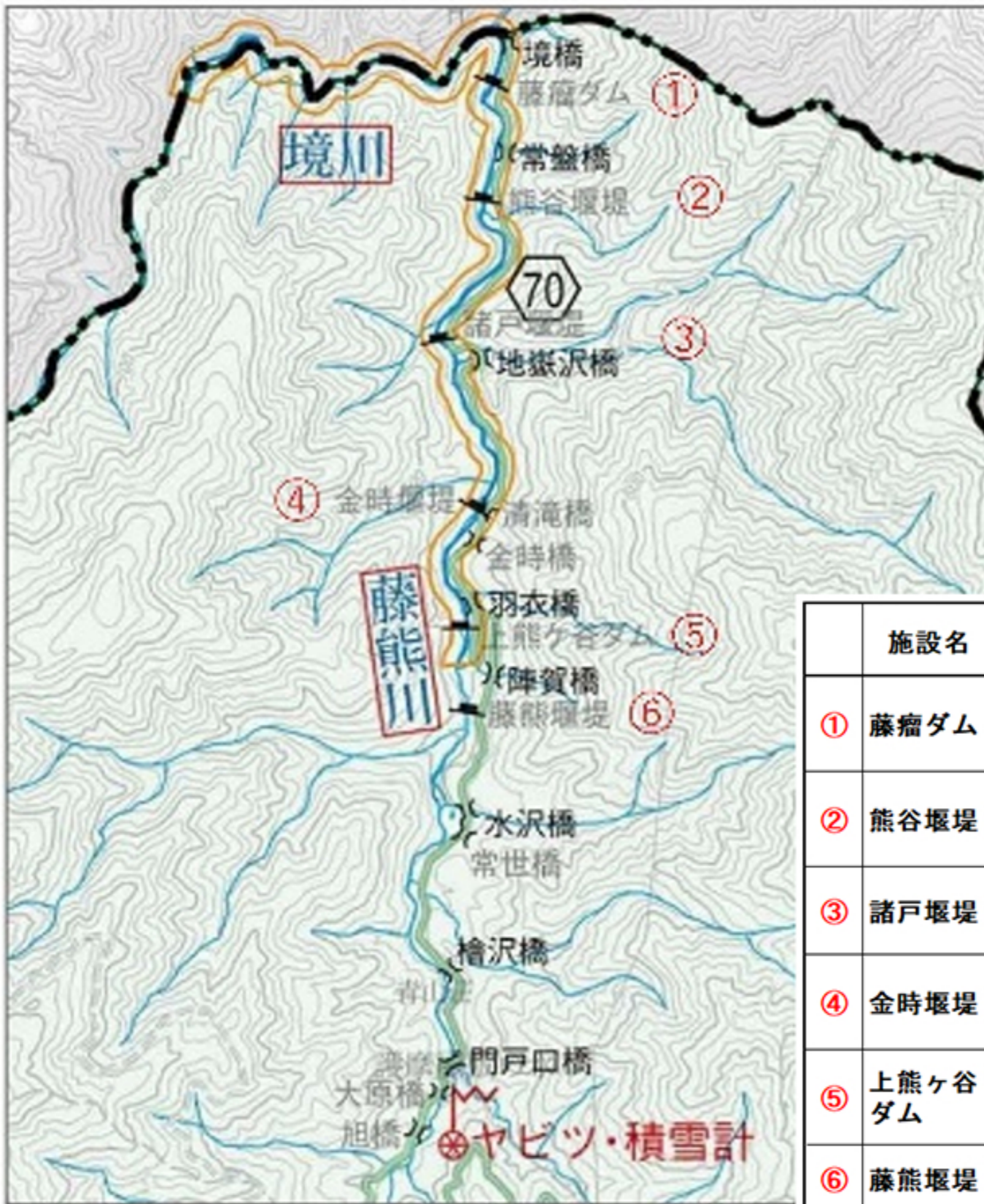
図8 藤熊川の砂防施設一覧図
