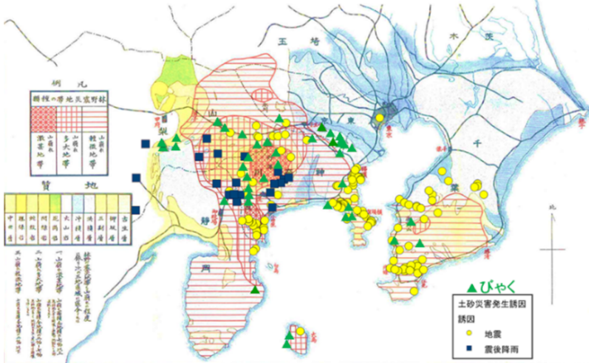
図8 関東地震による林野被害区域「山崩れ地帯」概況図と関東地震による土砂災害地点 井上（2013）に伊豆大島を追記，▲びやくの地点を追記（井上，2014，相原・井上（2016）
