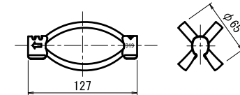
スペーサー S=1/3 SK85 (SK5) 電気めっき
