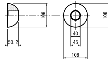
球面台座 S=1/5 FCD500-7 溶融亜鉛めっき (HDZT77)
