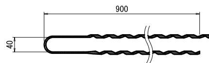
巻付グリップ S=1/5 φ12用-900 亜鉛アルミ合金めっき
