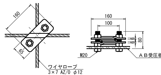
アンカークリップ S=1/5 SS400 溶融亜鉛めっき (HDZT49)
