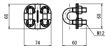
クロスクリップ S=1/3 SS400 溶融亜鉛めっき (HDZT49)
