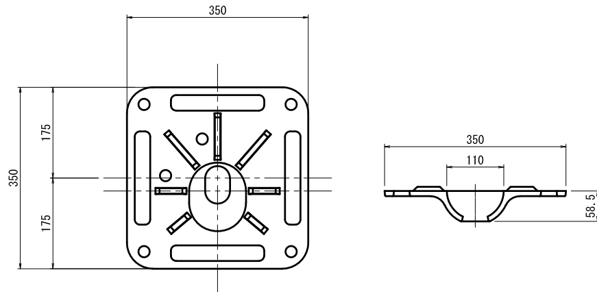
AB受圧板 S=1/5 FCD500-7 溶融亜鉛めっき (HDZT77)
