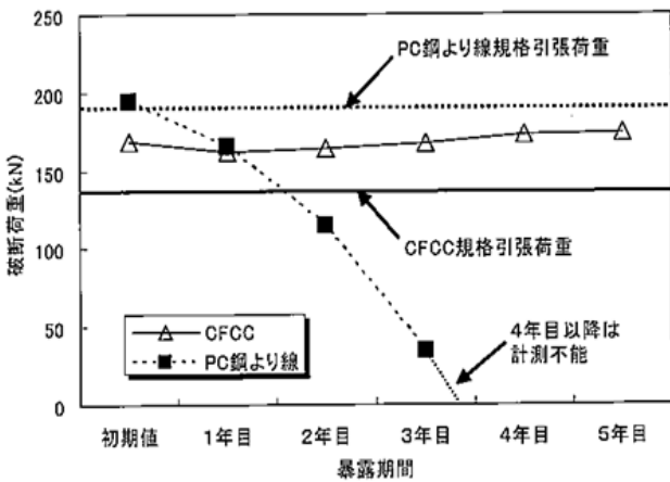
図-2 試験体の強度変化 (屋外暴露)
