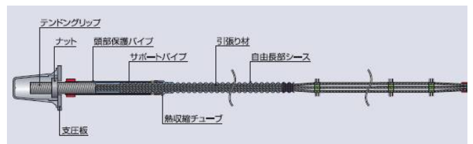
図-1 テンドン構造図
